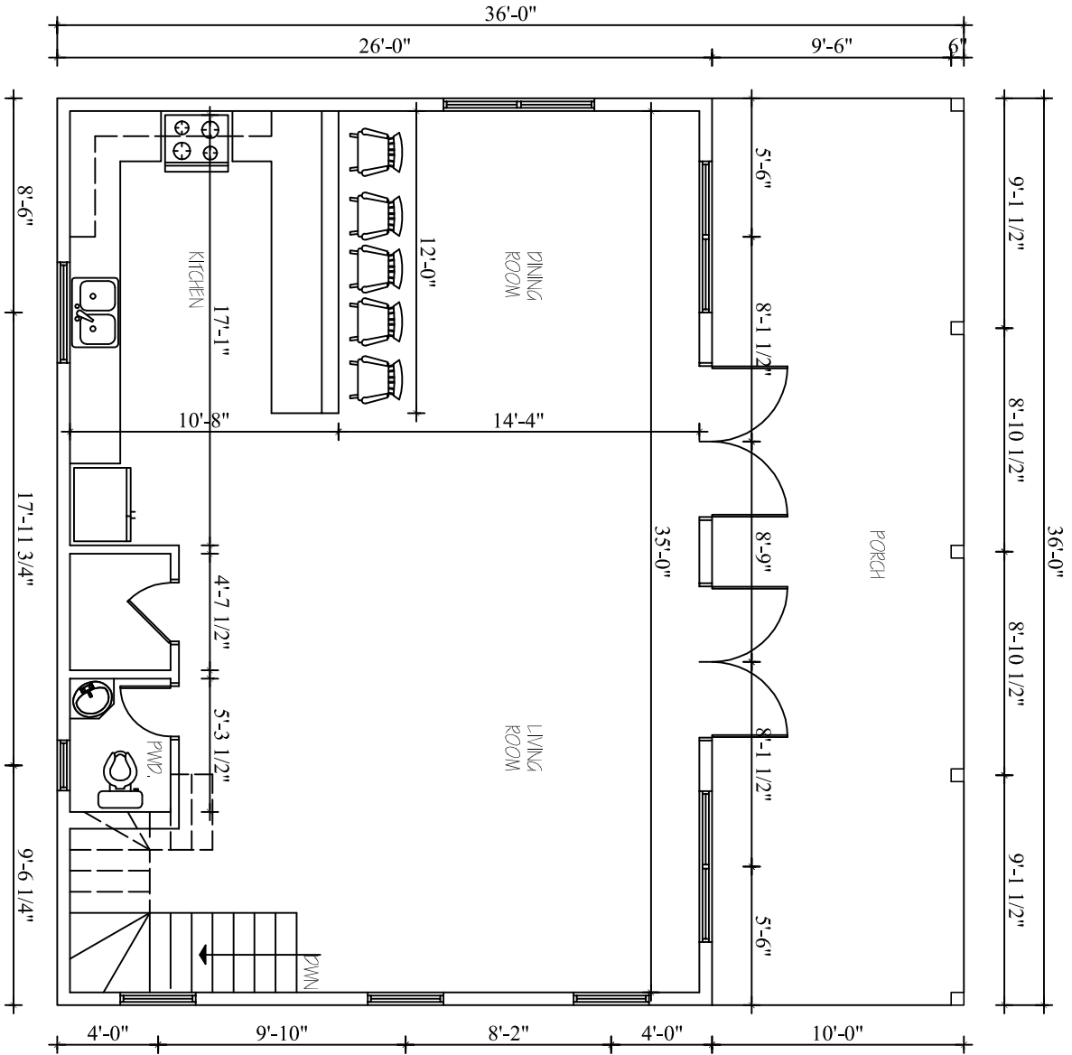
FIRST FLOOR PLAN SCALE: N.T.S.
